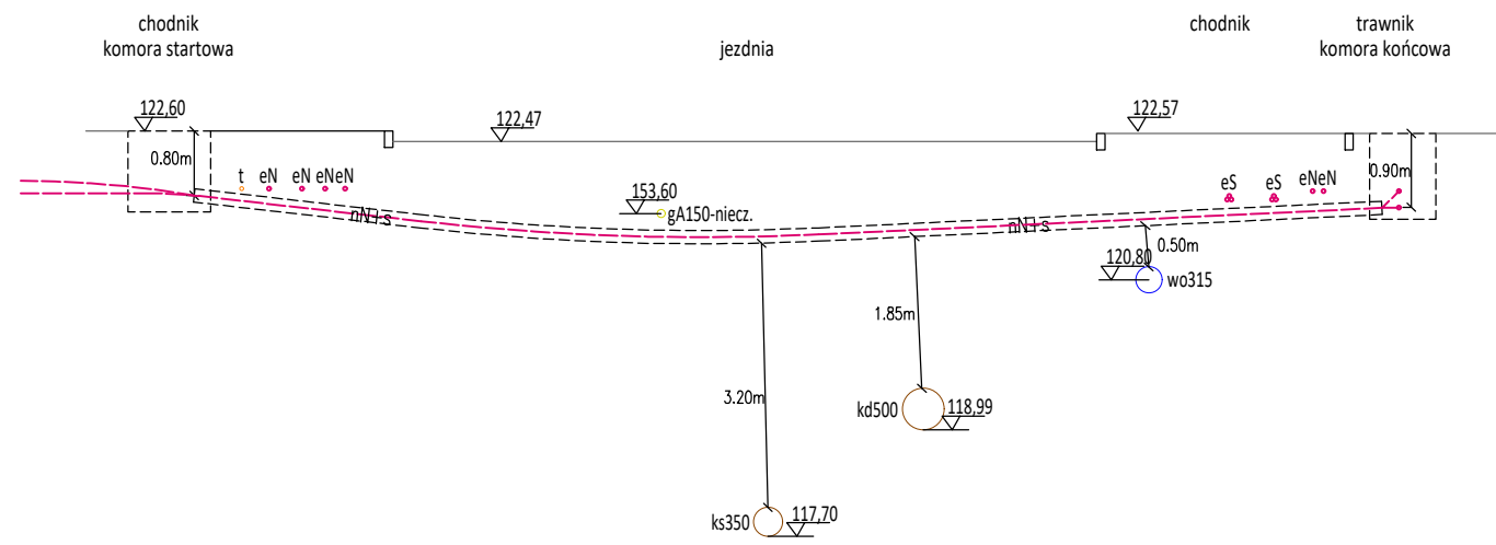
PROFIL B-B
