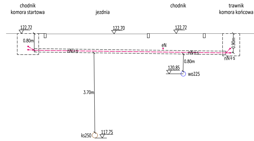
PROFIL C-C
