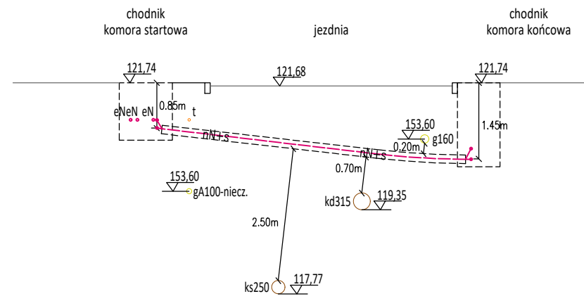
PROFIL A-A
